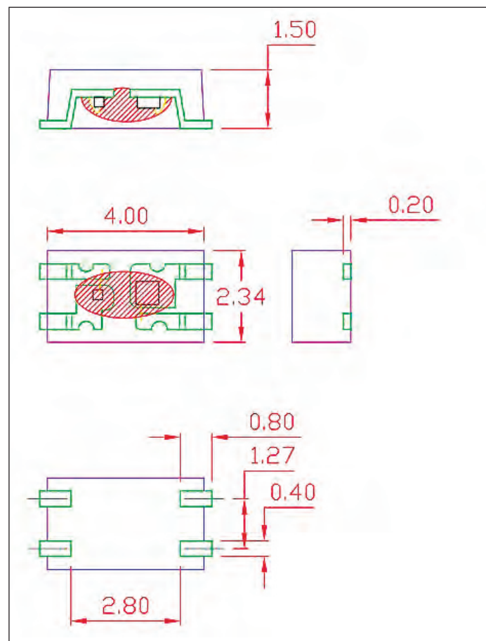
Bild 1: Lösung auf Basis von Leiterrahmentechologie
