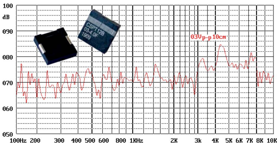
Piezo transducer frekvenciakarakterisztika (nincs beépített oszcillátor)
